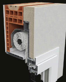
COFFRE 1/2 LINTEAU
