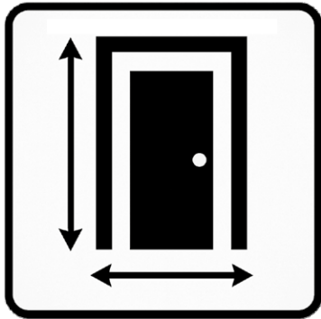
DIMENSIONS MAXI UN VANTAIL (POSE EN APPLIQUE) DOS DE DORMANT : H 2390 x L 1120 mm TABLEAU : H 2360 x L 1060 mm
