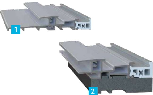
OPTION 1 BAVETTE DE SEUIL À CLIPPER Disponible en finition anodisée ton inox ou noire, elle est utile sur certains chantiers pour une finition parfaite.
